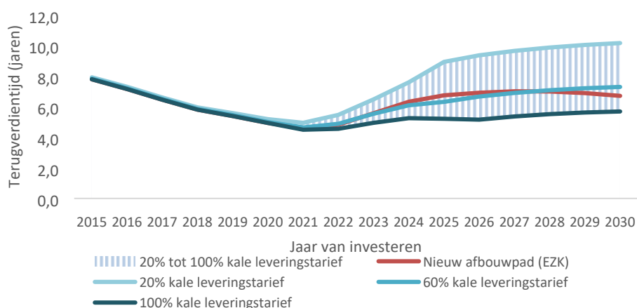
Figuur 1. De terugverdientijd van zonnepanelen voor referentiewoning bij het nieuwe afbouwpad (zoals voorgesteld door EZK) en bij het alternatieve voorstel van marktpartijen binnen de bandbreedte.
